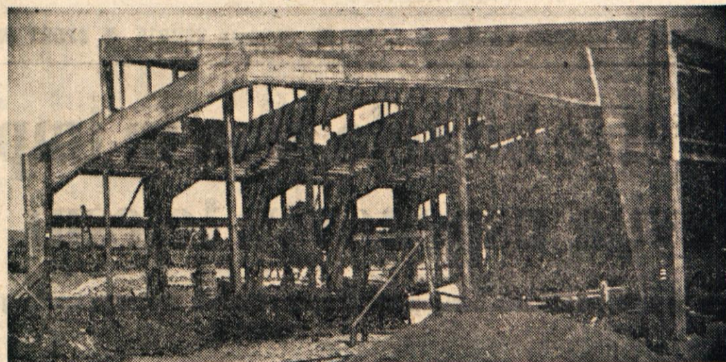
Betonski skelet nove NOVOLESOVE tovarne v Straži
