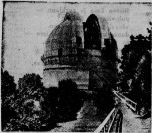
Sodobna zvezdarna — okno v vsejmirski daljine
