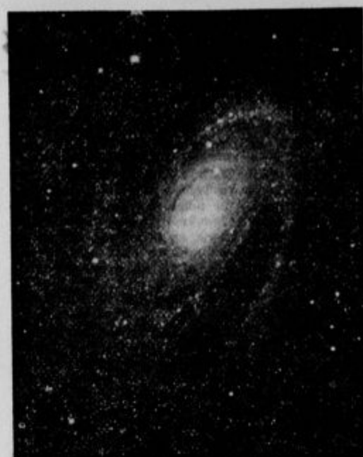
Spiralna meglica v Velikem vozu
