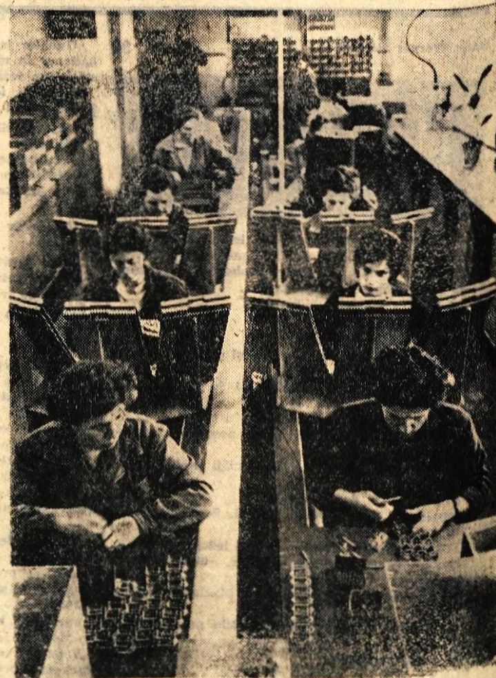
Vsaki 15 sekund na tem tekočem traku izdelajo v Lipnici po številčnik za števec
