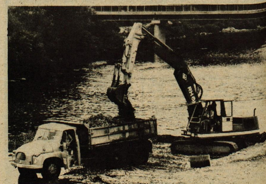
V Megradovi temeljni organizaciji združenega dela »Gradles« Medvode uporabljajo za nasipe material, katerega po dogovoru z Vodno skupnostjo Ljubljana-Sava črpajo iz reke Sore. Obenem s tem tudi čistijo strugo in držijo stalni vodostaj reke Sore.
