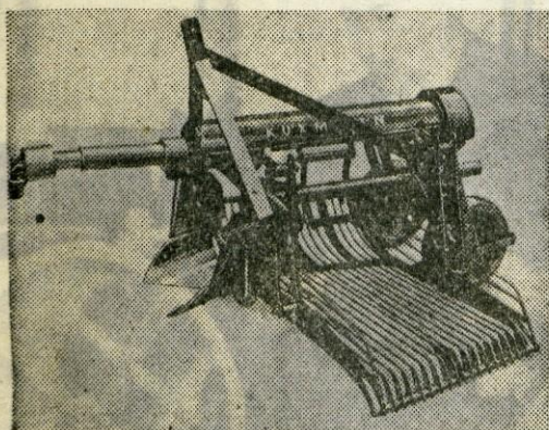
KUXMANN — izkopalnik za krompir
