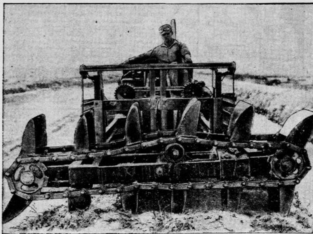
Česa bi potrebovali na svetu namesto topov in plinskih bomb? Dosti takšnih poljedelskih strojev, kakršen je gorenji, ki ga je izumil neki Američan. Ta stroj izravna, preorje in prevlači ozemlje, preko katerega gre in ustvarja idealna poljska tla.
