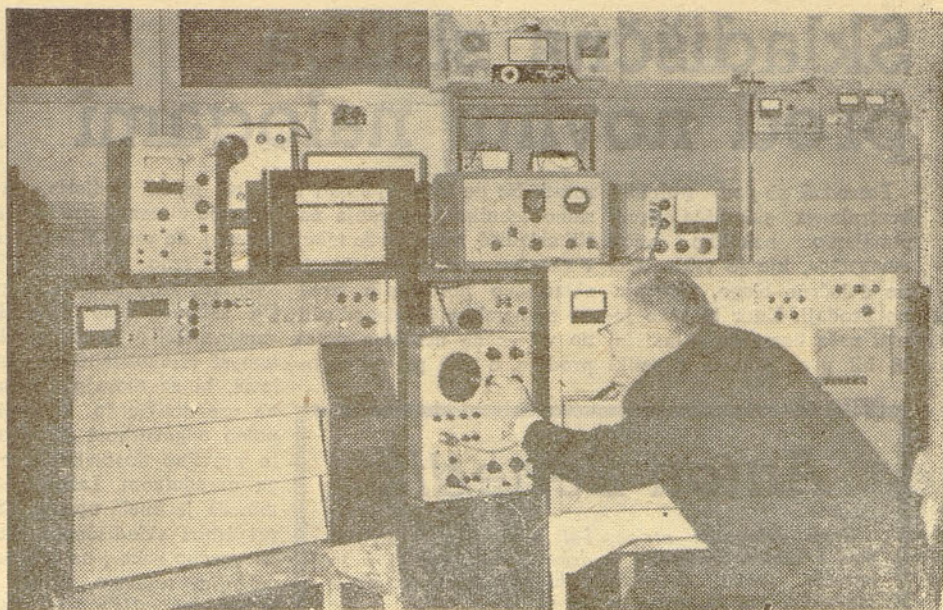
V prostorih »ELES« v Ljubljani je bila pretekli teden javna demonstracija prototipa nove telekomandne naprave, ki jo je izdelala skupina strokovnjakov APV — zavoda za avtomatizacijo pod vodstvom inž. Erna Petriča (na sliki)
