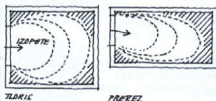
PREDDOR DNEVNE SVETLOBE V PROSTOR SKOZI OKNO
