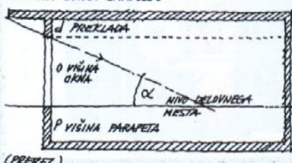
ZUNANJA OVIRA (NAPUŠČ)
