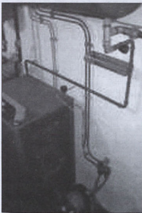
Primer namestitve ampule v kurilnici
