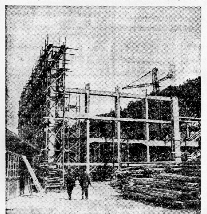
Sošanjska termoelektrarna — Pogled na gradbišče strojnice za novo termoelektrarno v Sošanju
