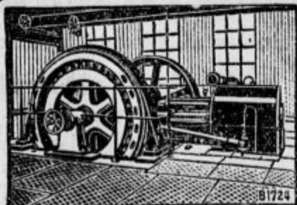
LANZOVE vročeparne Lokomobile z naravnost vezano Dynamo.
