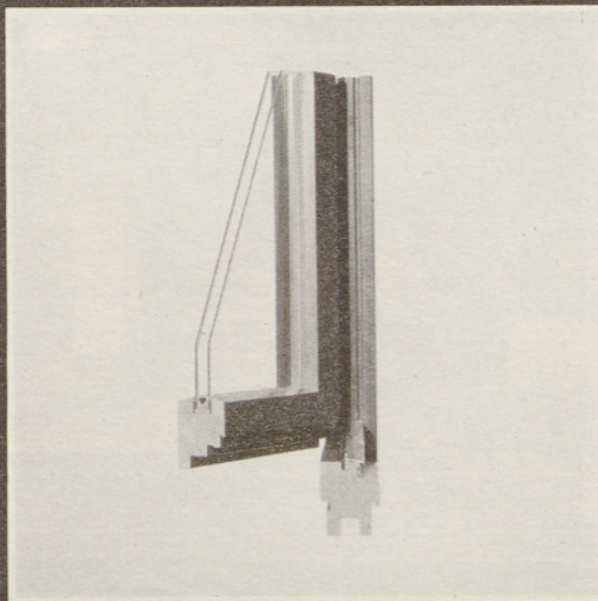
Prerez okna s termoizolacijskim steklom
