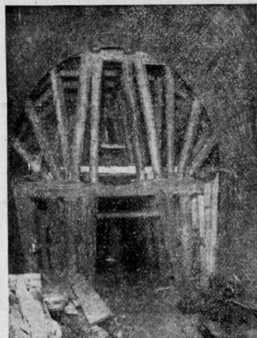
V ospredju betoniran prstan, v ozadju mogočna lesena konstrukcija, ki drži ogrode, za katerim bodo začeli betonirati nov betonski obroč
