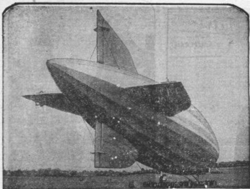
Nemci, ki so bili že pred in med vojno mojstri v gradbi vodljivih zračnih ladij, so zopet zgradil zračnega velikana, ki nakriljuje vse dosedanje. — Desno: Nova velika zračna ladja L. Z. 127 na prvem poletu.
