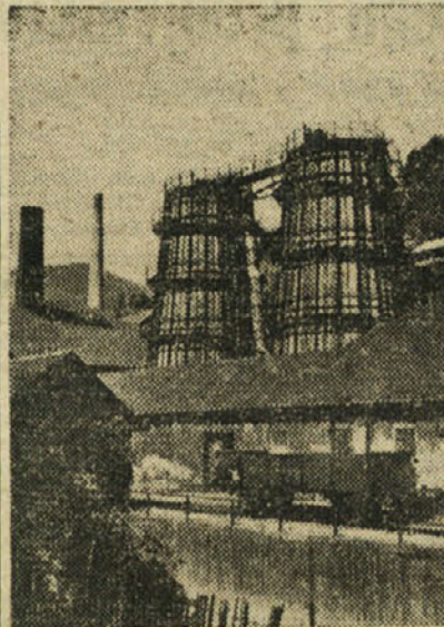
Obrat žveplene kisline
