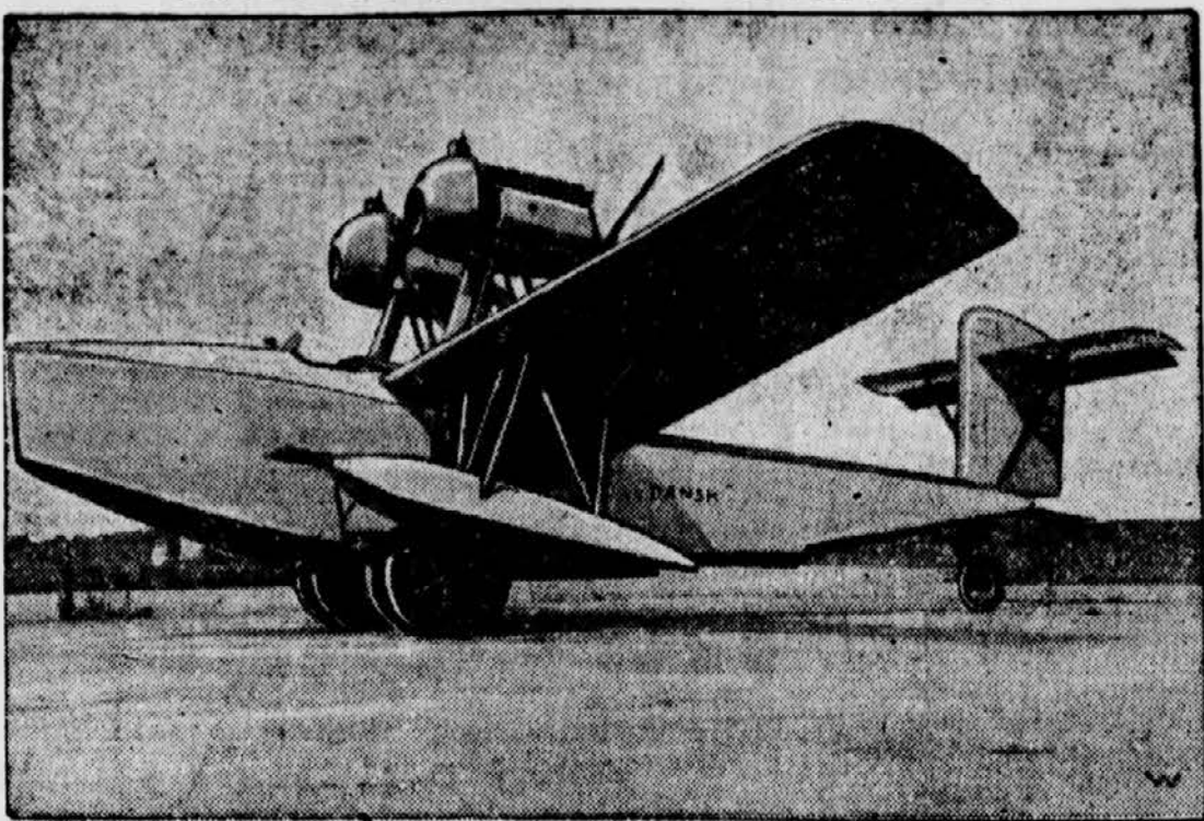
Das Flugboot „Robbe“ zum Landtransport auf Räder gesetzt.
