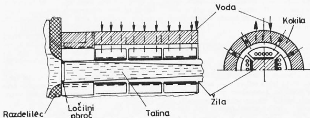
Slika 4. Sekundarno hlajenje za kokilo s pritisnjenimi grafitnimi ploščami
