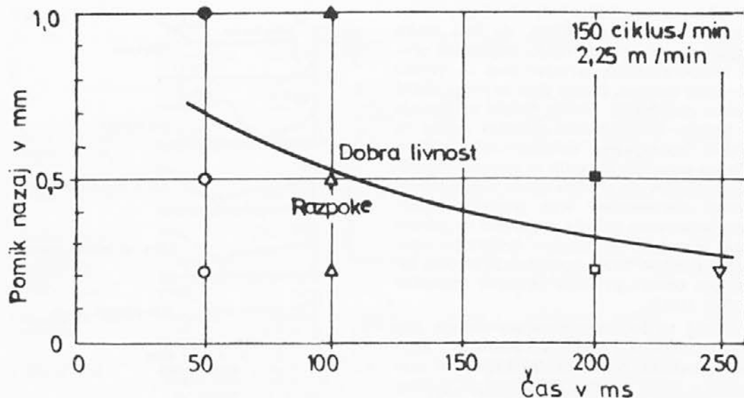
Slika 7. Preizkušeni program za nastavitve pomika nazaj in pavze pri načinu vlek — pomik nazaj — pavza (150 ciklov/min., hitrost litja 2,25 m/min.)
