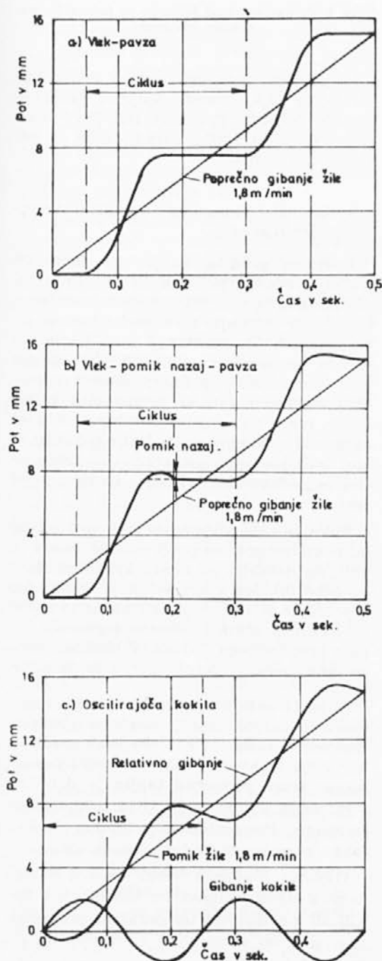
Slika 5. Različni načini pomikanja žile pri HCC postopku
