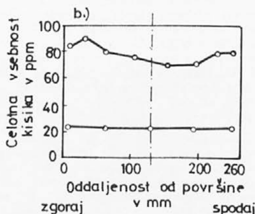
Slika 17. Nesimetrična porazdelitev makro vključkov in kisika v horizontalno kontinuirni gredici
