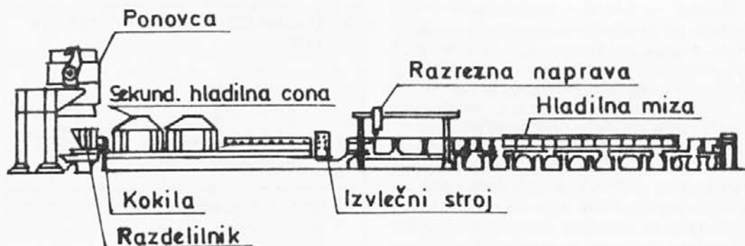
Slika 2. Shema HCC naprave
