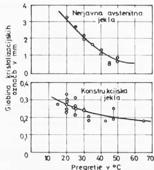
Slika 12. Vpliv pregretja na globino hladnega zvarca
