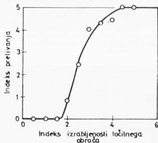
Slika 14. Soodvisnost med prelito površino in izrabo ločilnega obroča
