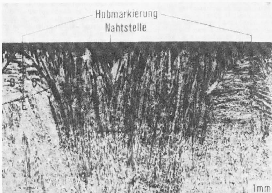
Slika 10. Strjevalna struktura vzdolž pomika gredice, jeklo Č 4578 (PK 19), Ø 96 mm
