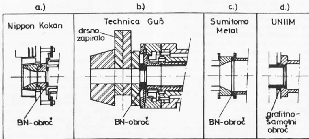
Slika 3. Različna izvedba povezav med kokilo in razdelilnikom
