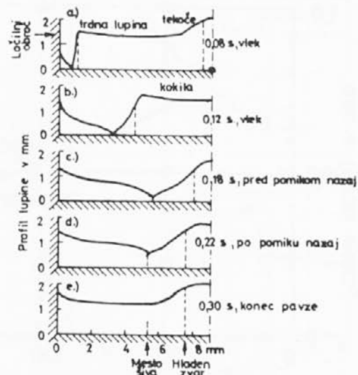
Slika 6. Strjevanje v kokili med izvlačenjem po načinu vlek — pomik nazaj — pavza po sliki 5 b
