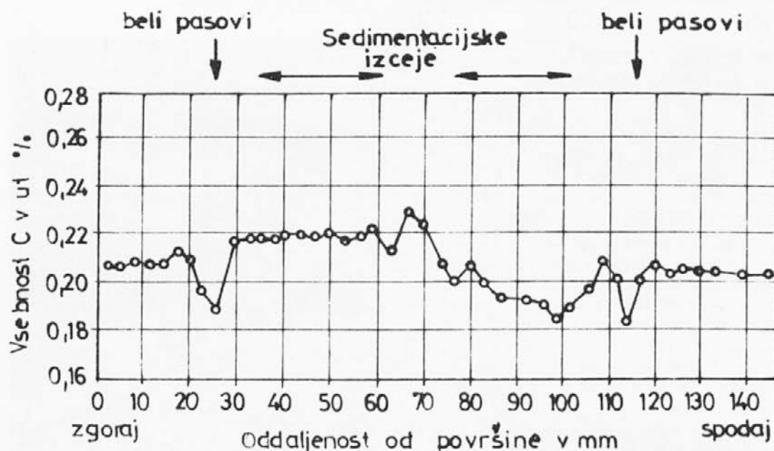
Slika 16. Vsebnost C po preseku HCC žile Ø 150 mm mešane z elektromagnetnim mešalcem
