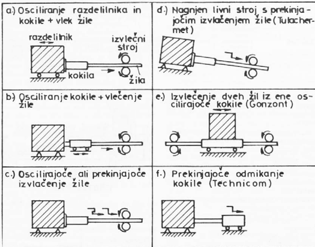
Slika 1. Shematični prikaz razvoja HCC naprav
