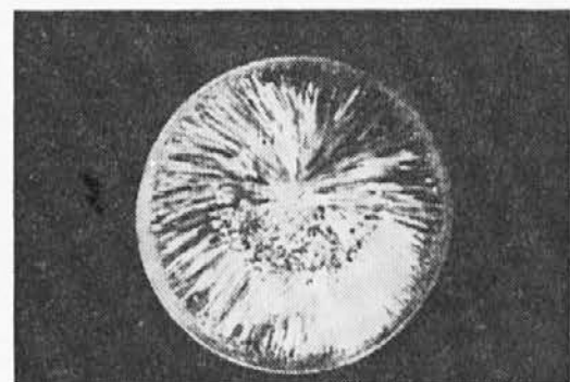
Slika 15. Gredica Ø 150 mm z nesimetrično razporejenimi globuliti, jeklo Č 4972 (PK 924)
