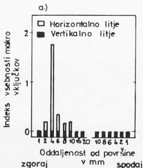
Slika 17. Nesimetrična porazdelitev makro vključkov in kisika v horizontalno kontinuirni gredici
