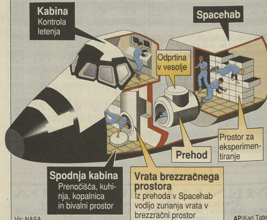
Prerez vesoljskega plovila Endeavour
