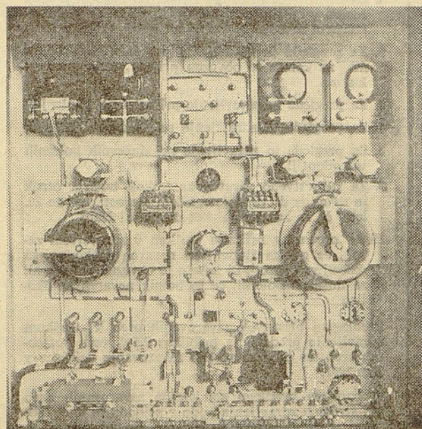
Stikalna plošča — izdelek učencev poklicne šole Iskra Kranj, spada med vsakoletni šolski program praktičnega pouka
