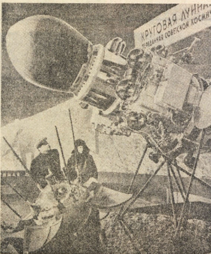
Medel avtomatične postaje «Luna 9» na razstavi v Moskvi. (Iz «Pravde»)
