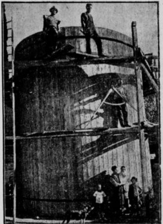
Velika kad, ki je bila izdelana v Skofji Loki za papirnico v Goricanah. Kad ima 106.164 litrov vsebine. Za njo so porabili 19 m 3 mecesnovega lesa in 970 kg železa.
