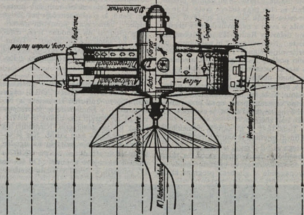
Podroben prikaz bivalnega kolesa po ing. Potočniku
