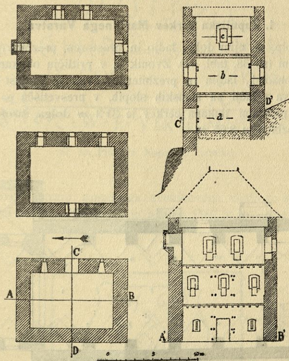
Sl. 37. Tlorisi pritličja in dveh nastropij ter preseka po črtah A B in D C Kebelske graščine. — Merilo 1 : 400.
