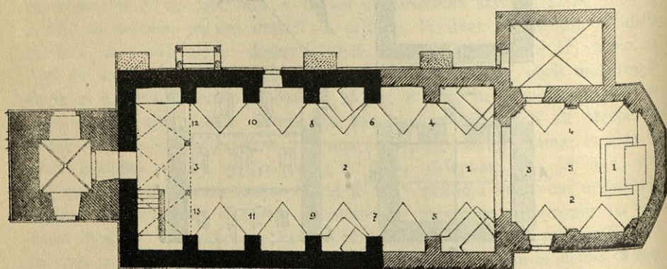
Sl. 38. Prihova. Tloris župnijske cerkve. Merilo 1 : 300.
