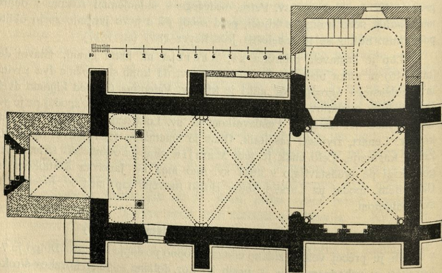
Sl. 52. Špitalič. Tloris župnijske cerkve. Merilo 1 : 200.
