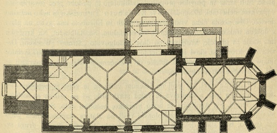
Sl. 30. Župnija Čadram. Tloris podružnice sv. Barbare. Merilo 1 : 300.
