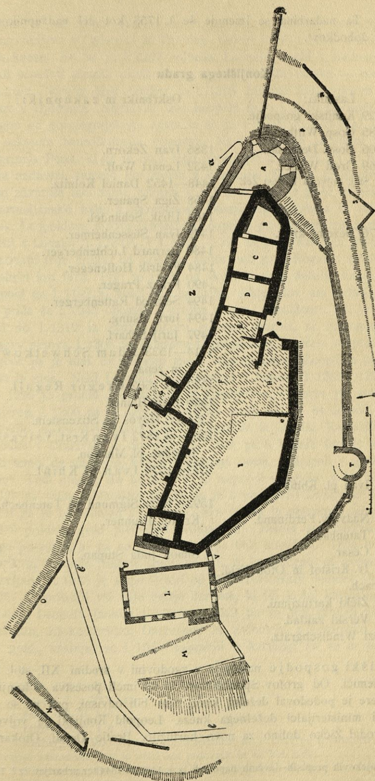
Sl. 7. Konjice. Tloris konjiškega gradu.
