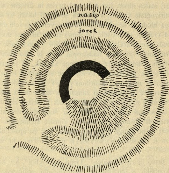
Sl. 36. Tloris Kebelskega gradu. Merilo 1 : 400.
