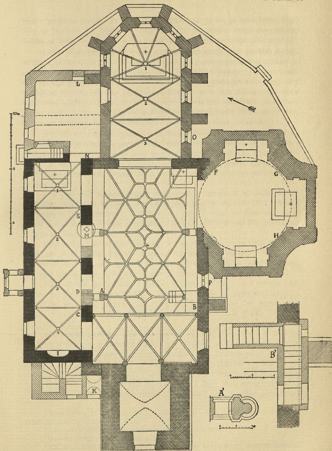
Sl. 4. Konjice. Tloris nadžupnijske cerkve sv. Jurija.
