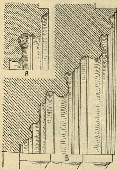
Sl. 57. Špitališ. Presek čelnih okrožic pri stranskih (A) in glavnih (B) cerkvenih vratih.
