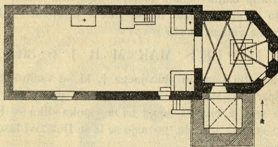
Sl. 35. Župnija Kebel. Tloris podružnice sv. Lenarta. Merilo 1:300.
