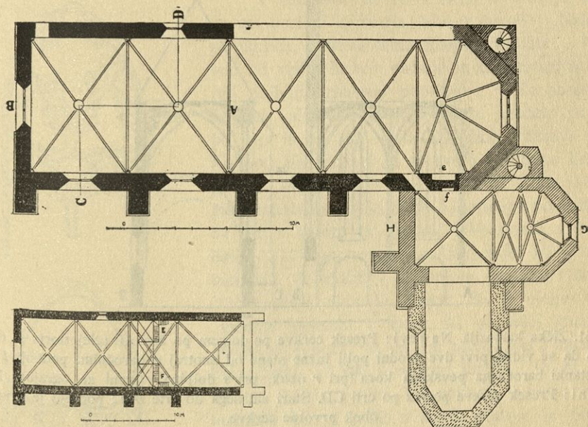
Sl. 60. Žička kartuzija. Zgoraj: Tloris cerkve. Črkam AB in CD odgovarjata preseka v sl. 61. Pri e je bil najbrž sedile. Ob desni: Tloris dvonadstropne kapele. Po črkah GH se je naredil presek v sl. 66. Pri f je bil ali vhod v grobnico, ali pa (predno so napravili sedile na tem mestu) zveza s prezbiterijem. — Merilo 1 : 300.
