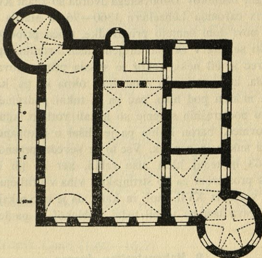
Sl. 8. Tloris graščine Golič pri Konjicah. Merilo 1 : 300.
