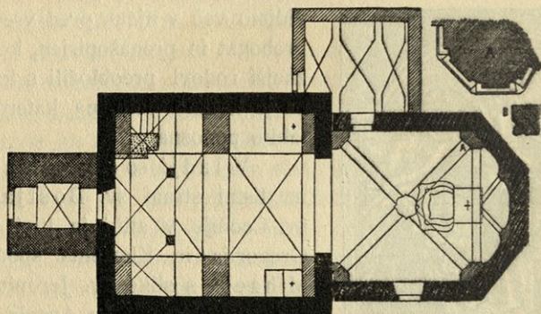
Sl. 42, Prihova. Tloris podružnice sv. Jošta. (Presek gotskega podboja B spada k glavnim vratom pod zvonikom). Merilo 1 : 300.
