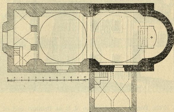
Sl. 13. Zreče. Tloris podružnice M. B. na Brinjevi gori. Merilo 1 : 300.
