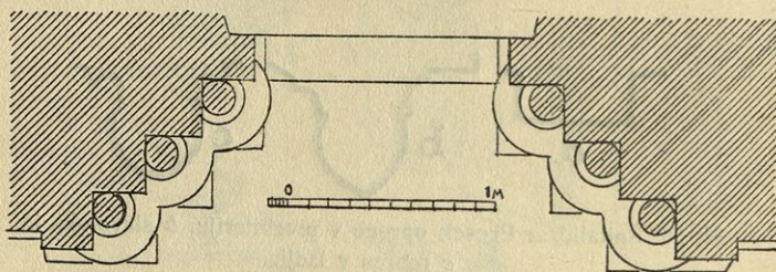
Sl. 56. Špitalič. Tloris podbojev glavnih cerkvenih vrat.
