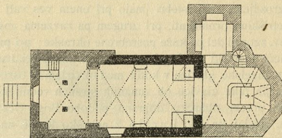
Sl. 16. Zreče. Tloris podružnica sv. Martina. Merilo 1 : 300.
