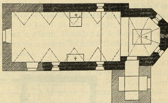
Sl. 25. Resnik. Tloris podružnice sv. Jakoba. Merilo 1 : 200.
