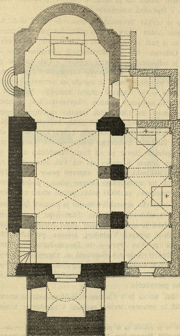
Sl. 27. Čadram. Tloris stare župnijske cerkve. Merilo 1 : 200.
