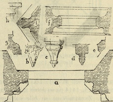
Sl. 70. Žička kartuzija. Podrobnosti od grobne kapelice. a Presek podbojev. b in c Dve konzoli za rebresa. e Presek rebres spodaj in d presek na vrha oboka. f Presek okna. g . Presek podnožnega okrajka zunaj kapele, h pa venčni zidec od zunaj in i presek „podpornika.“
