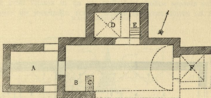
Sl. 20. Jamnik. Tloris nekdanje kapele sv. Pankracija. Merilo 1 : 200.
