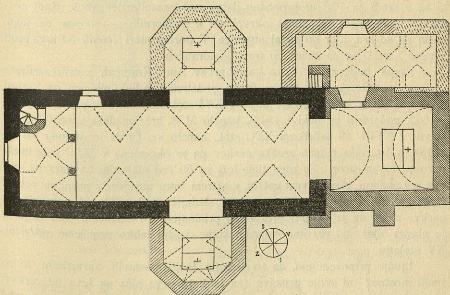
Sl. 11. Zreče. Tloris župnijske cerkve sv. Ilja.
