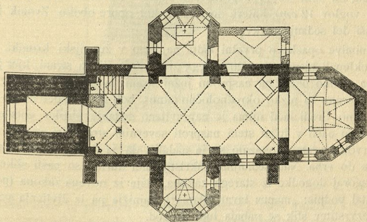
Sl. 23. Sv. Kunigunda. Tloris župnijske cerkve.
