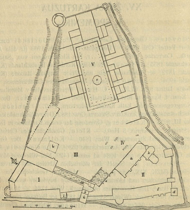
Sl. 59. Tloris Žiške kartuzije. I—V. Dvorišča. a Cerkev. b Dvonaestropna kapela. c Pokopališka kapela. d Zunanja kapela. e Klet. f Hodišče. g Prehod iz dvorišča I v II. h Stolp nad potokom. i Sedanji vhod. k Krnica za vodo. l Stanovanja. 1
