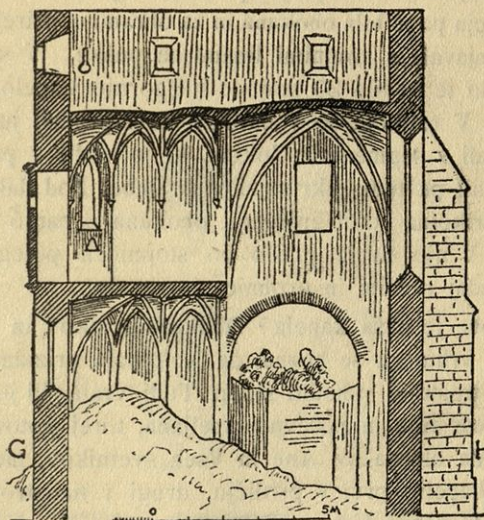
Sl. 66. Žička kartuzija. Presek dvonadstropne kapela po črti GH v tlorisu sl. 60.
