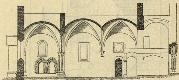
Sl. 53. Špitalič. Podolžni presek župnijske cerkve (Po Grausu). Merilo 1 : 300.
