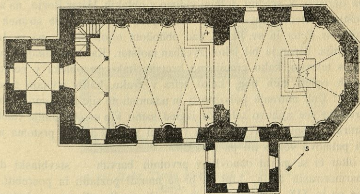
Sl. 15. Zreče. Tloris podružnice sv. Neže na Goliki. Merilo 1 : 300.
