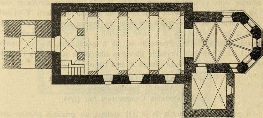
Sl. 28. Župnija Čadram. Tloris podružnice sv. Mohorja.
