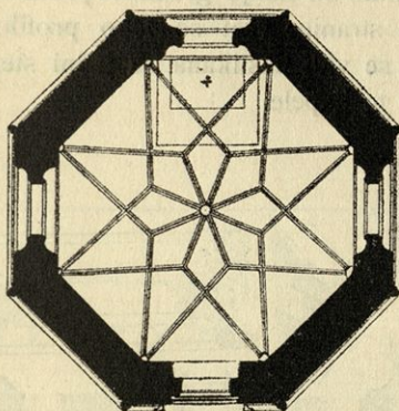
Sl. 69. Žička kartuzija. Tloris grobne kapelice. Merilo 1 : 150.
