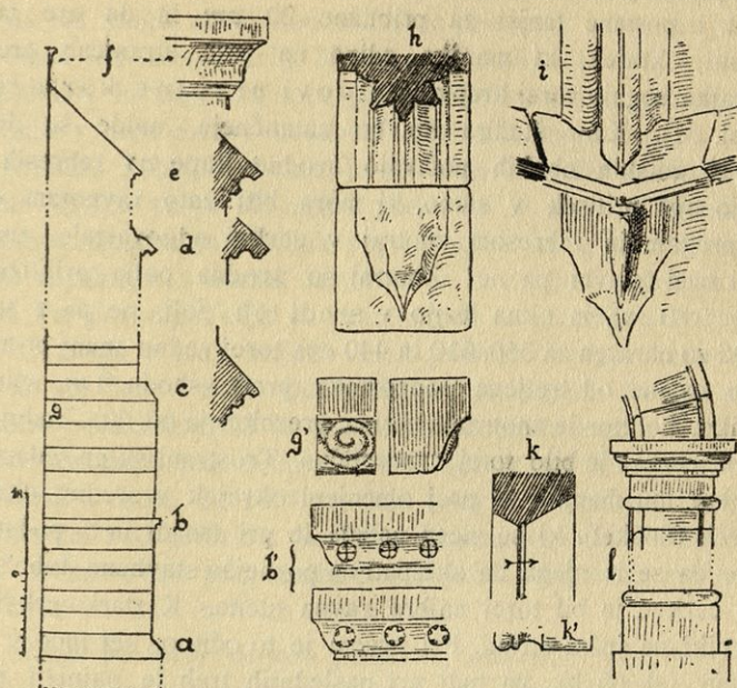
Sl. 65. Žička kartuzija. Podrobnosti iz cerkve. a-f sprednji južni sklepnik z ob strani v večjem merilu narisanimi okrajki, b' romanski okrajek, g' konzola v legi g . h Presek in spodnji konec služnikov v ladji. i Spodnji sklep služnikov v trostranem sklepu (ta detajl po Haasu). k Presek romanskega okna in k' profil enega kamna, ki se je pri tem oknu porabil kot gradivo. l Podnožek in glavica baročnih pilastrov v južni cerkveni steni.
