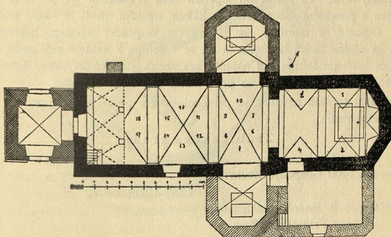
Sl. 46. Loče. Tloris župnijske cerkve.
