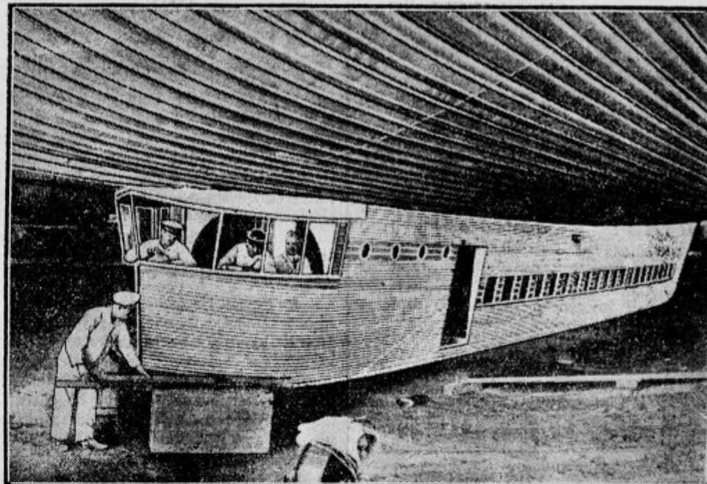
Novi angleški popolnoma kovinasti zrakoplov »City of Glendale«, ki ga ne žene bencin, kot Zepeline, temveč para. S pomočjo na poseben način konstruiranega propelerja, more mirno stati v zraku, medtem ko potniki vstopajo in izstopajo. Slika nam kaže zrakoplovovo gondolo.
