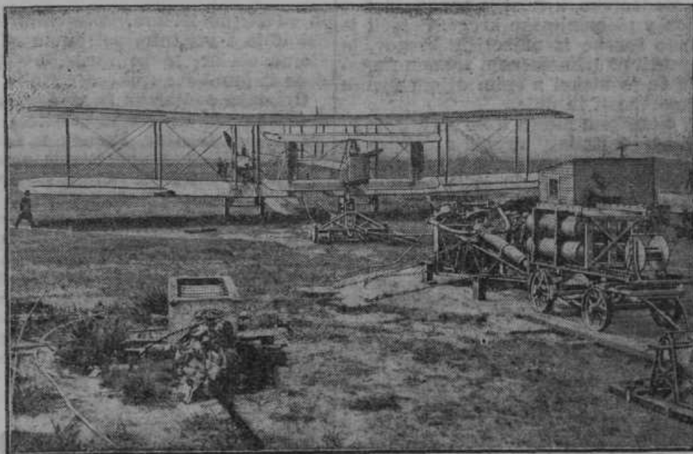
Stroj za odlet letal. Doslej so uporabljali stroje za odlet aeroplanov na velikih parnikih. Sedaj so ustvarili na Angleškem stroj za odlet letal na suhem. Namen novoizumljenega stroja je, si prihraniti letališče. Slika nam kaže trenutek, ko odsune stroj v zrak letalo.
