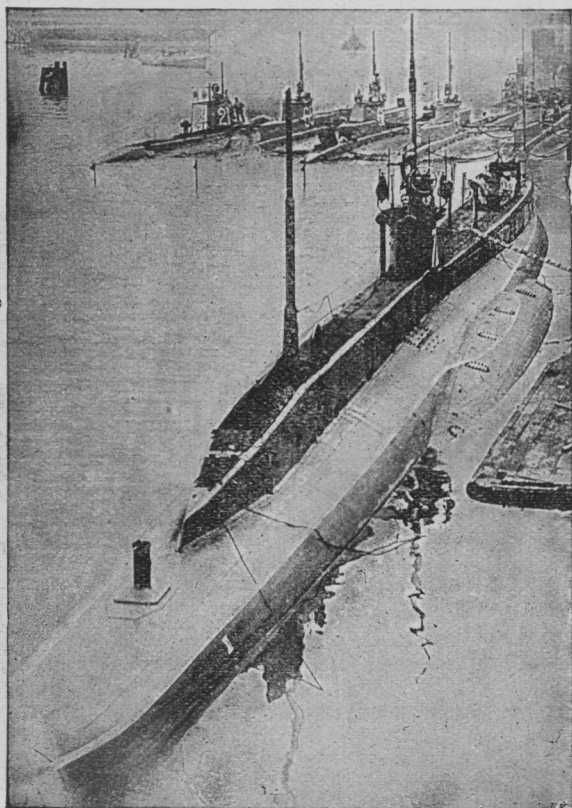
Angleški podmorski čoln, največji na svetu, iznajdba inženjera Thorneta Nordenfeldta. Čoln je okoli 3,5 m širok, 12,5 m dolg in do 3 m globok; ima dvojne vrste strojev za petrolej in za plin za plovbo v vodi; potaplja se z akumulatorji in elektromotorji; pod vodo more plavati tri ure s hitrostjo 9,2 vozla ter nad vodo s hitrostjo 12,1 vozla in strelja iz sebe torpede.
