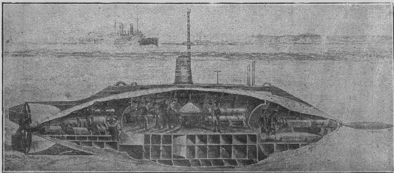
Podmorski čoln. Nemški torpedni čoln „U 9“ je uničil te dni sam 3 velike angleške križarice. Spredaj (na desnt) torpedo pripravljen, zgoraj moli nad morskno gladino cev „oko“ čolna.
