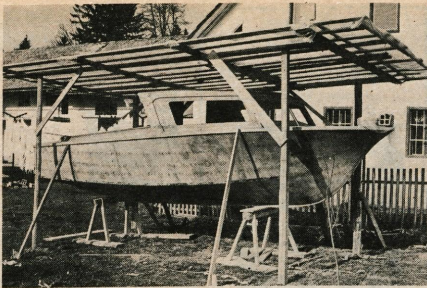
Babičev čoln, dolg 6,65 metra in širok 2,10 metra čaka, da ga bo konstruktor dokončno opremil. — Foto: F. Perdan
