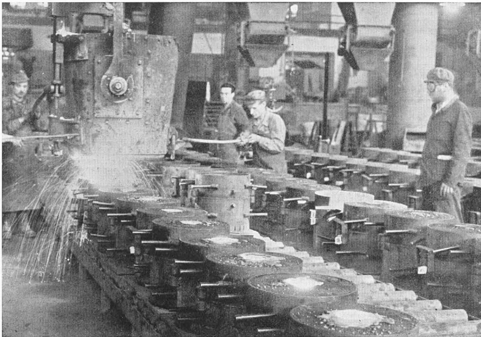
STROJNA LIVARNA — Ulivanje serijske litine
