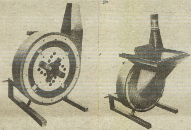
Drobilec z avtomatsko dozirno napravo, za katerega je dipl. ing. Vlado Mihalič dobil nagrado in priznanje (bila je edina v občini Ljutomer) za inovatorstvo.
