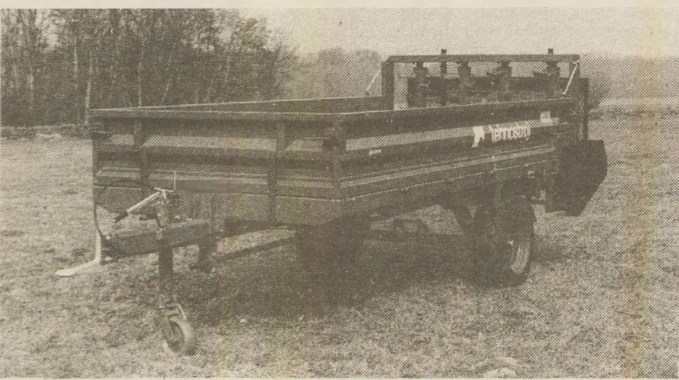
Trosilnik hlevskega gnoja, uporaben tudi kot prikolica za spravilo pridelkov
