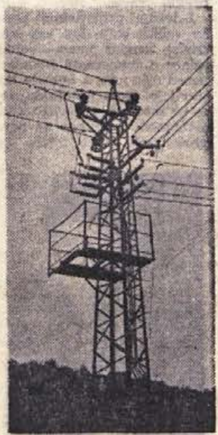
Transformatorska postaja na Brveh bo prav kmalu začela pošiljati elektriko na Stojanski vrh in v okoliške vasi. Prav takšno transformatorsko postajo so postavili tudi v Bušci vasi
