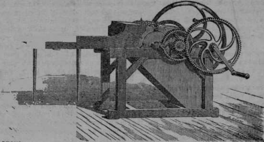
huttleworth-ova ročna mlatilnica. (fig. I.)
