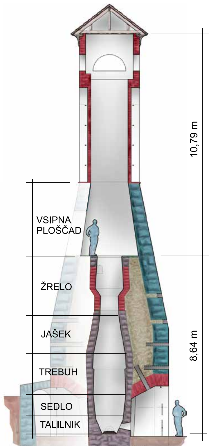
Prerez plavža v Železnikih, razdeljen na posamezna območja, kjer se je opravljala postopna redukcija (taljenje) železa iz rude v grodelj. Risba: Bojan Rihtaršič
