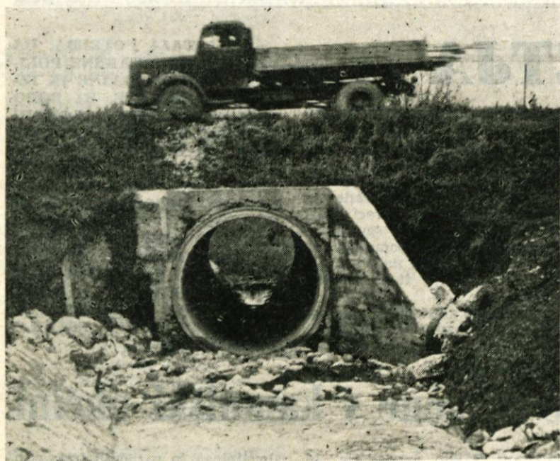
Razbremenilnik na Pšati v Mostah so začeli čistiti. Pravijo, da bo treba povečati tudi propust pod cesto Moste-Brnik, ki je sedaj »ozko grlo« tega razbremenilnika.
