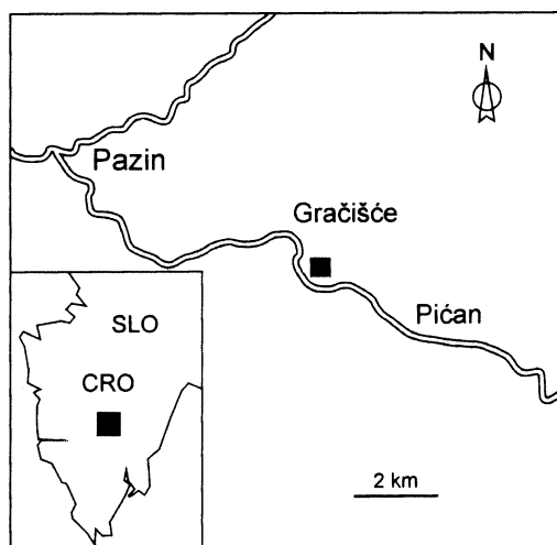
Sl. 1 Položaj najdišča rakovice pri Gračišću na Hrvaškem
