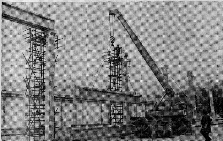
Montaža primernih nosilcev
