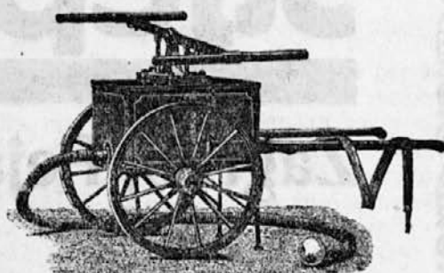
Dvokolna brizgalnica, podvojeno brizgajoča 180—200 \frac{2}{\text{min}} .
