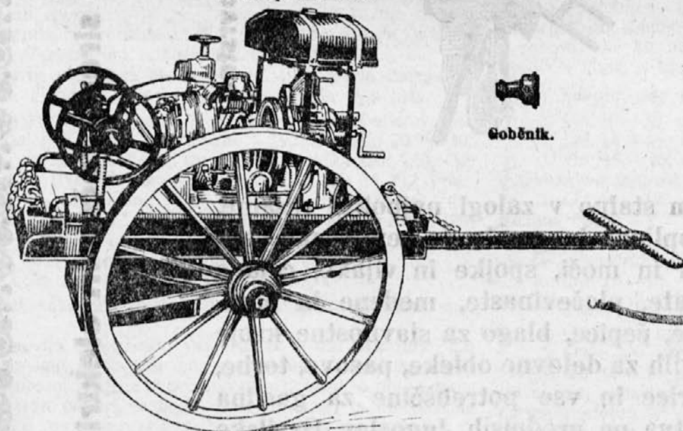
Motorna brizgalna tipa „MB 2“.
