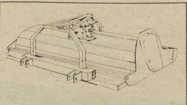
MULČER CM 140 CIMOS delovna širina: 1400 mm pogonska moč: 30 kW delovna hitrost: 4—8 km/h teža: 440 kg
