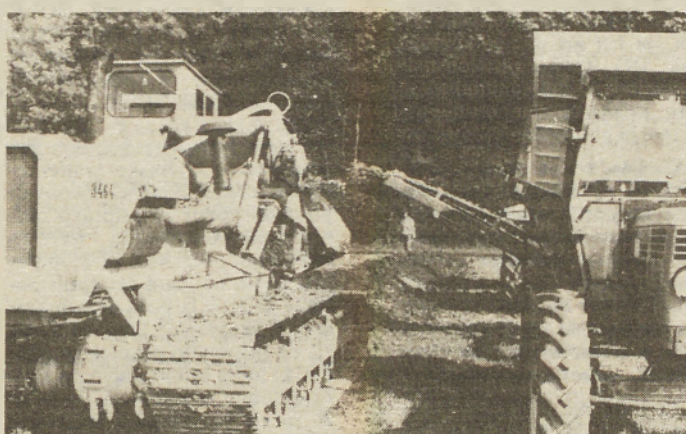
Kopanje drenažnih jarkov. Ko stroj izkoplje kanale in obenem položi drenažne cevi, jih drugi takoj zasuje.
