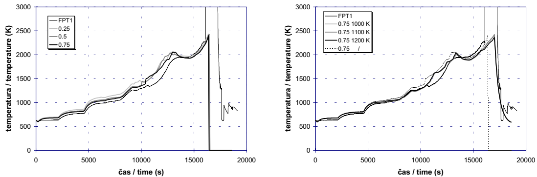
Sl. 8. Temperatura goriva v zunanjem obroču sredice na višini 300 mm za različne sevalne izmenjalne količnike (levo) in za različne temperature zapiranja parnih rež (desno)
