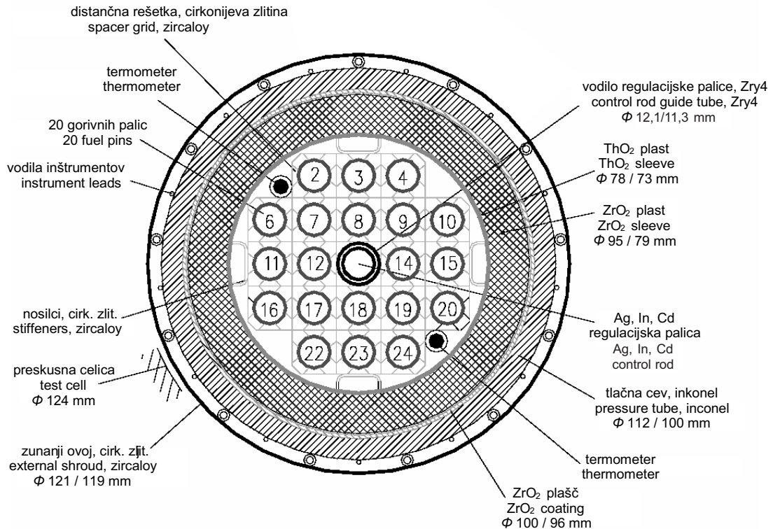
Sl 2. Prečni prerez FPT1 reaktorske posode z gorivnim svežnjem Fig. 2. Radial configuration of the FPT1 bundle
