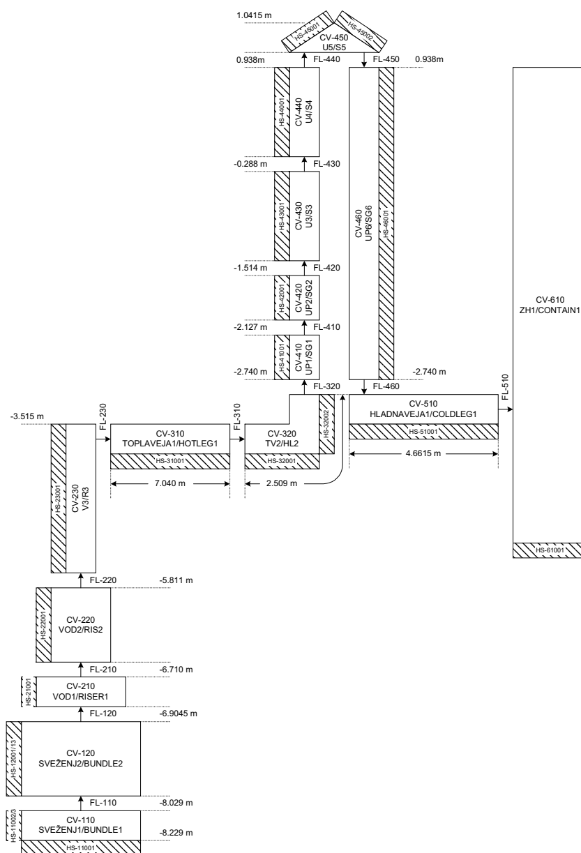
Sl. 4. Termohidrodinamična nodalizacija primarnega kroga in nodalizacija toplotnih teles Fig. 4. Thermalhydraulic and heat structure nodalization of the bundle and circuit
