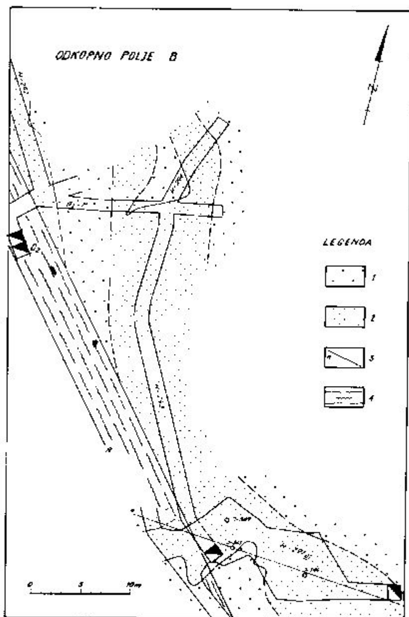
Sl. 17. Odkopno polje B, talninska rudna plast 1 sivi peščenjak, 2 ruda, 3 prelom, 4 prelomna zona Fig. 17. Stopping area B, the footwall ore bed 1 Gray sandstone, 2 Uranium ore, 3 Fault, 4 Fault zone
