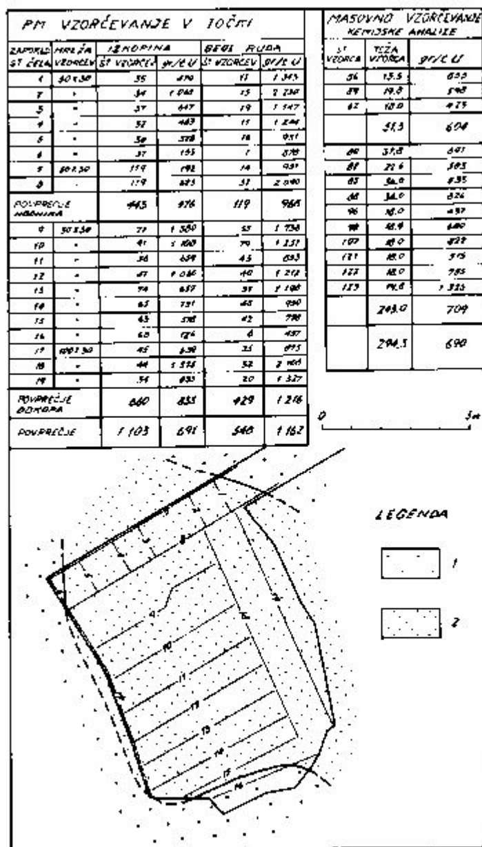
Sl. 23. Odkop O 1 -P, dokumentacija eksploatacijskega raziskovanja 1 sivji peščenjak, 2 uranova ruda
