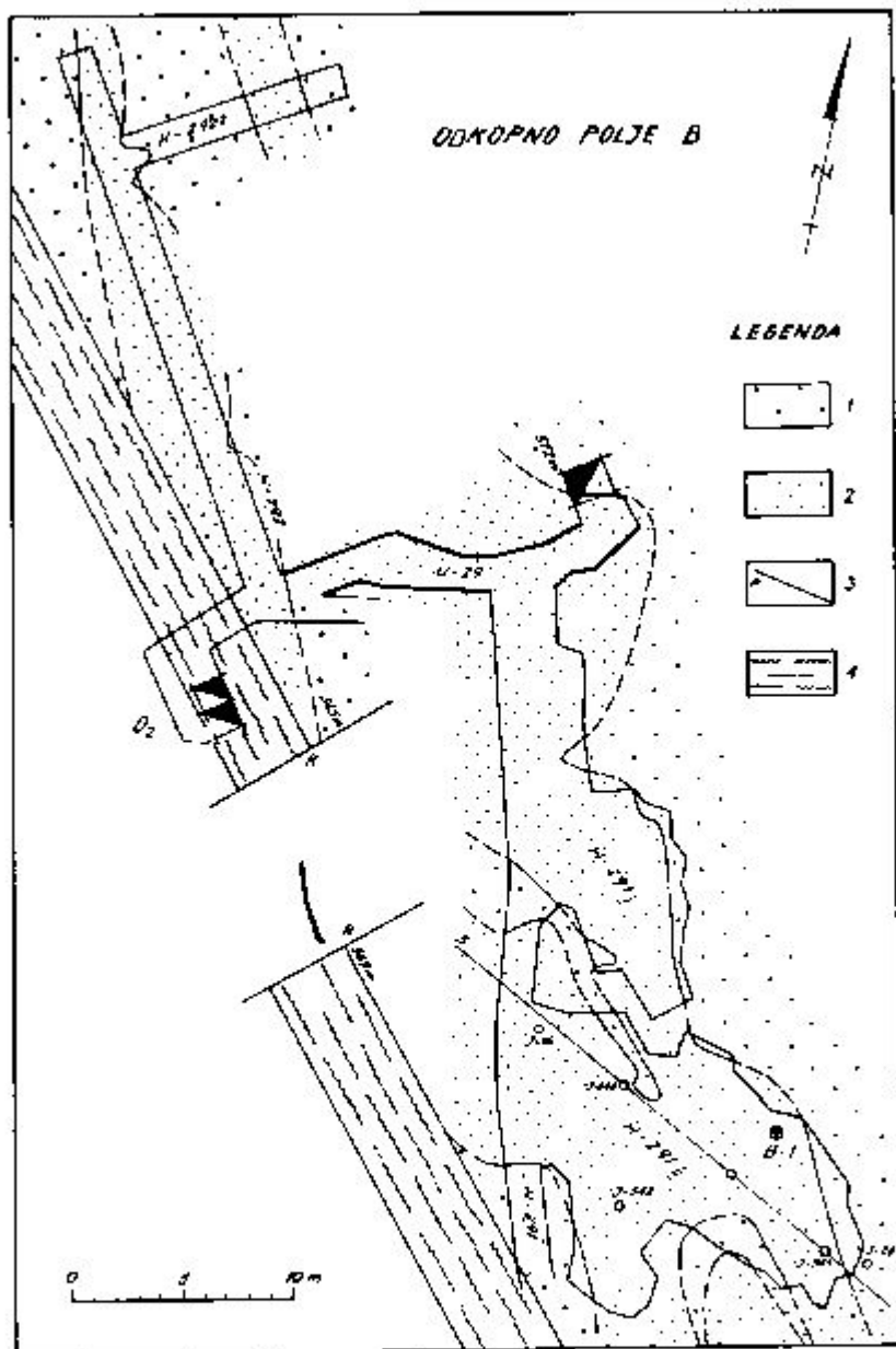
Sl. 15. Odkopno polje B, krovinska rudna plast 1 sivi peščenjak, 2 ruda, 3 prelom, 4 prelomna zona
