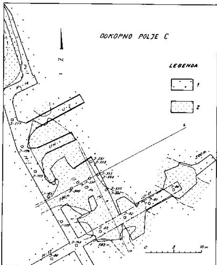
Sl. 19. Odkopno polje C
