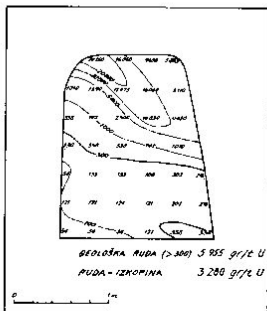
Sl. 10. Mreža točkovega radiometričnega vzorčevanja na čelu hodnika H-291. Gostota 30 × 30 cm
