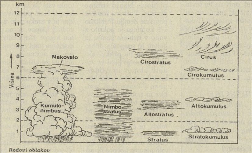
Slika prikazuje shematično razdelitev oblakov na rodove
