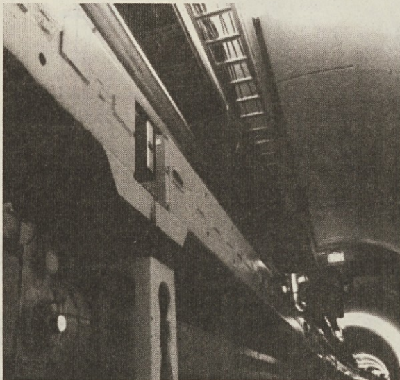
Tevatron - zgoraj je obročasta cev z navadnimi, spodaj pa cev trkalnika s superprevodnimi magneti.
