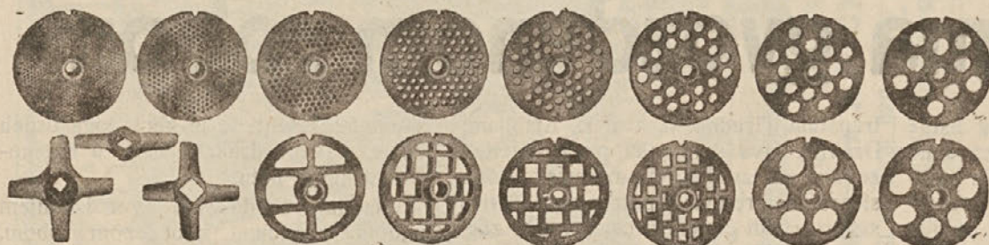
Ploče i noževi br. 5 do 32
