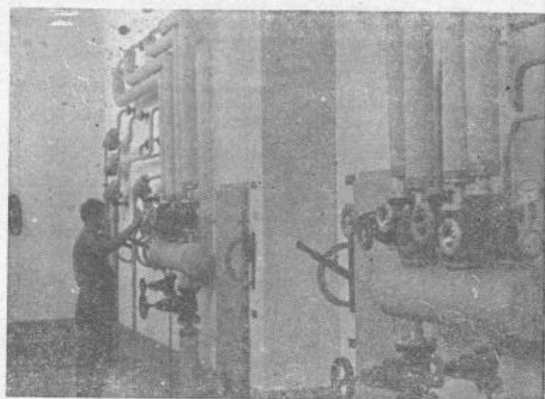
Komandni prostor v sušilnici za les — »Elanc, Begunje
