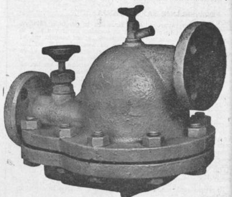
Kondenzni lonec za pritisk do 6 atmosfer
