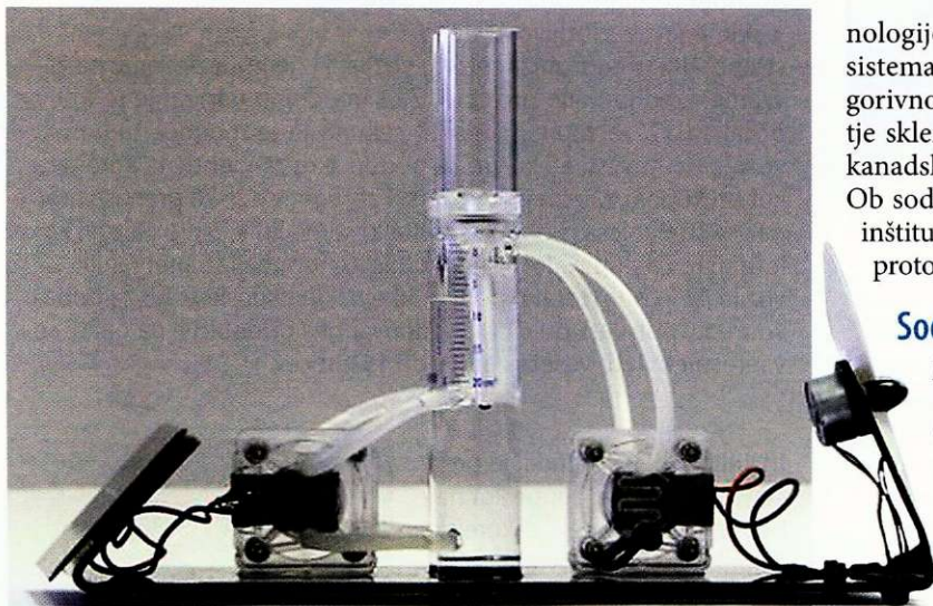
Prikaz delovanja gorivnih celic
