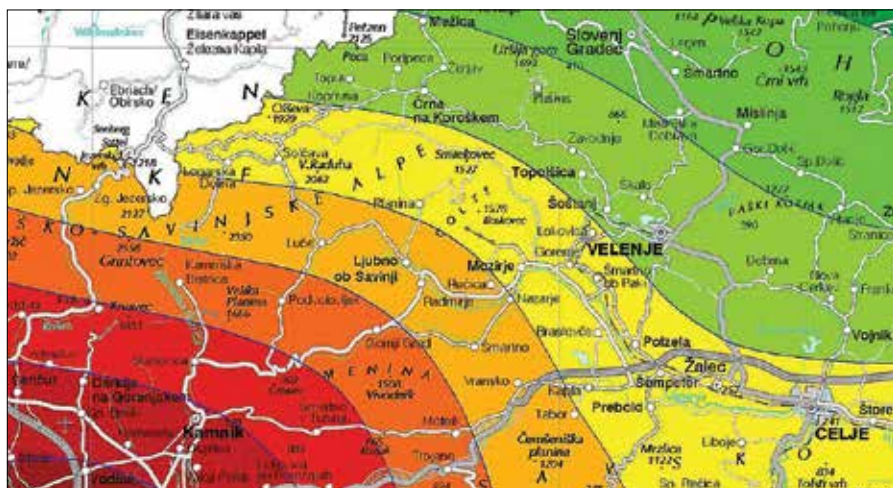
Izsek iz karte potresne nevarnosti Slovenije (Vir: ARSO Urad za seizmologijo)
