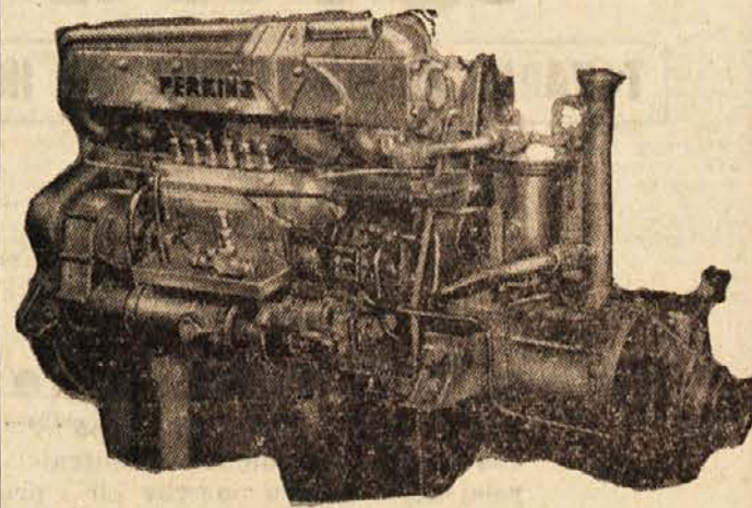
Tipa „56-M“ specialni ladijski motor
