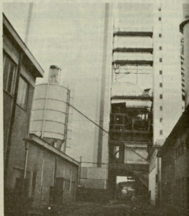
Zahodna stran bloka štiri v šoštanski termoelektrarni. Iz dimnika se že po poskusnem zagonu razžvepljevalne naprave vali čistejši dim, v katerem je predvsem para.
