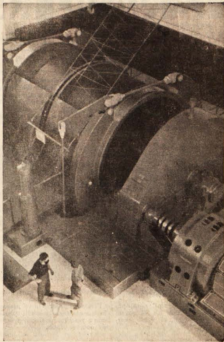
Naš fotoreporter se je na poti po Štajerskem ustavil tudi v Velenju, kjer je najbogatejši rudnik lignita v naši domovini. Bil je prijetno presenečen, ko je videl mogočne naprave novega jaška. Na sliki, ki jo je posnel, vidimo strojno ob izvoznem stolpu. Na novega leta bodo vse naprave montirane in takrat bo začel novi jašek obratovati.
