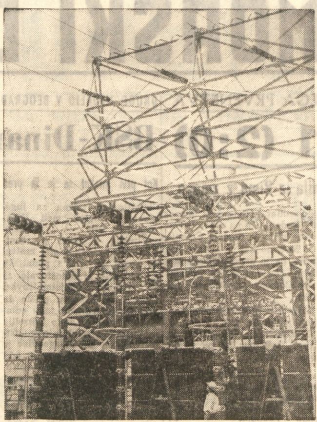
V tem labirintu izolatorjev in žic povečujejo napetost električnega toka iz velike sodobne elektrarne v Aliverju v Grčiji od 15.000 na 150.000 voltov
